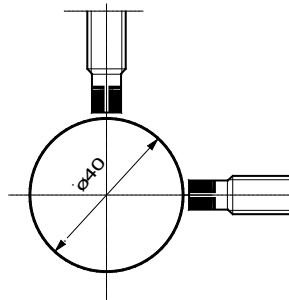
Abstand zur Wellenschulter Sensor parallel zu elektrisch leitfähigem Material Distance to shaft shoulder Sensor parallel to electrically conducting material Distance à l'épaule d'arbre Capteur monté en parallèle à un matériel conducteur
